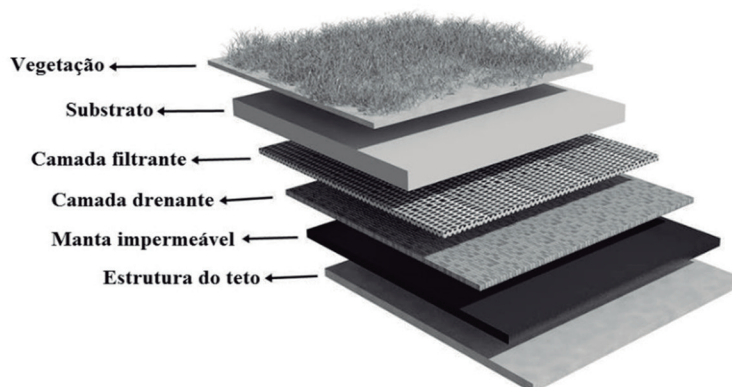
Figura 1 - Camadas obrigatórias do telhado verde
